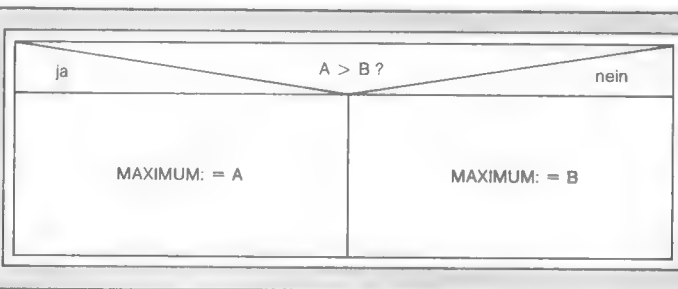
Bild 4. Struktogramm der IF-Anweisung mit ELSE-Zweig
